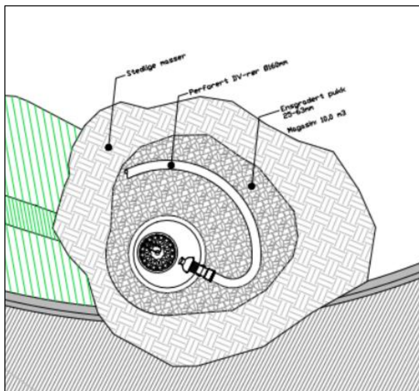
Figur 9 Eksempel på drensrør ut frå kum
