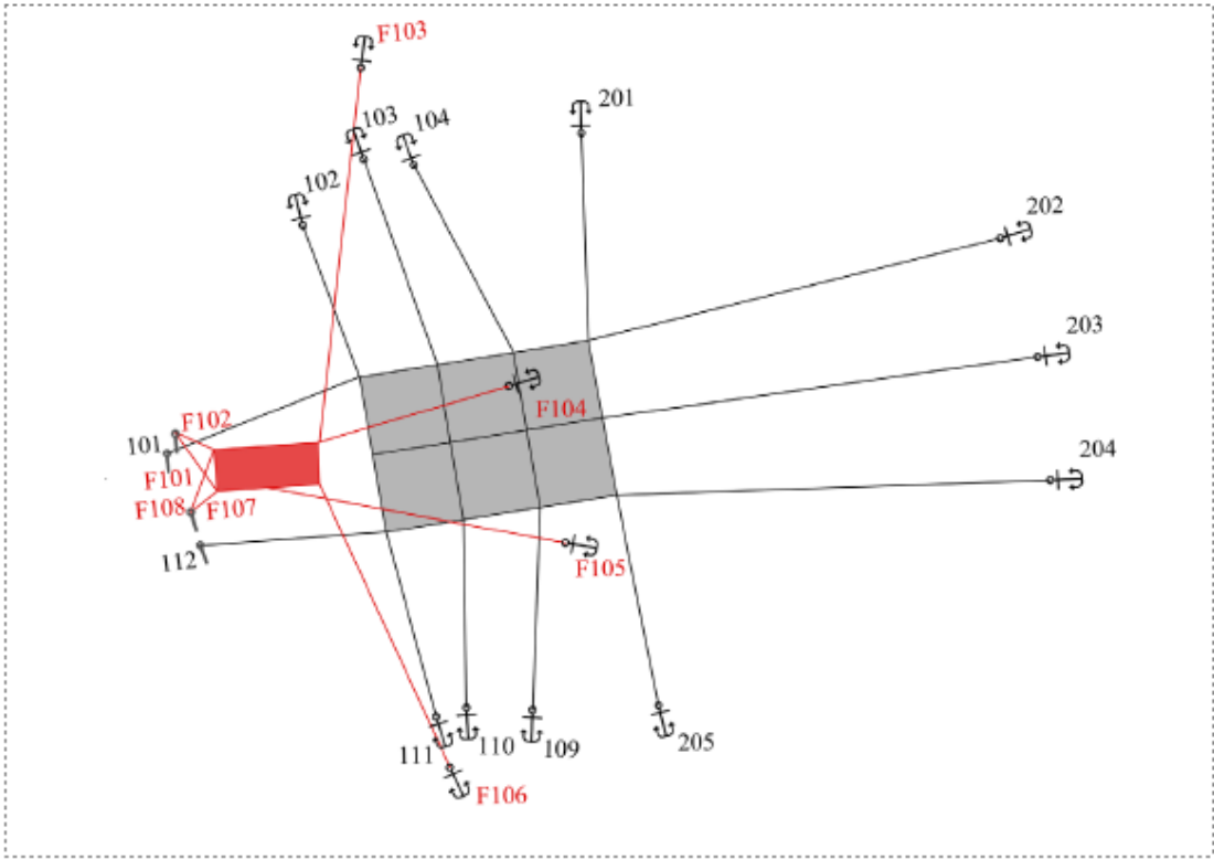
Figur 3. Anleggsforankring med nummerering av liner.
